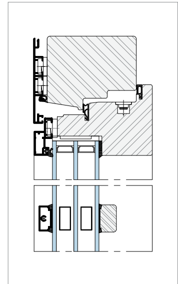
Aufgeklebte und abgedichtete Sprosse – 28 oder 36 mm (beispielhaft mit 3-fach Verglasung)
