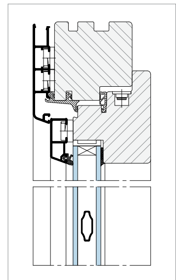
Sprosse im Scheibenzwischenraum 18 oder 26 mm (beispielhaft mit 2-fach Verglasung)
