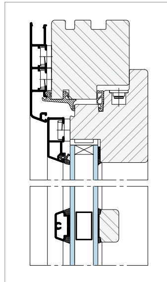
Aufgeklebte und abgedichtete Sprosse – 28 oder 36 mm (beispielhaft mit 2-fach Verglasung)
